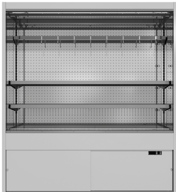
Longueur disponible (sans joues) : 625-937-1250-1875-2500 mm Epaisseur joue miroir / panoramique : 41 mm/unitaire
